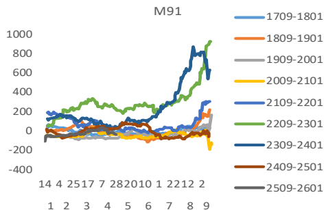
图 5: M91 价差
