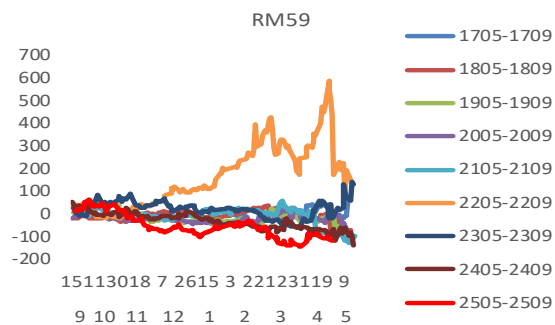
图 4: RM59 价差
