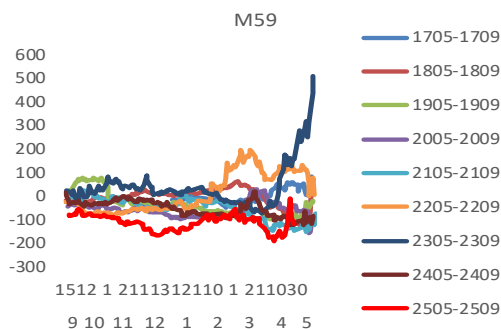
图 3: M59 价差
