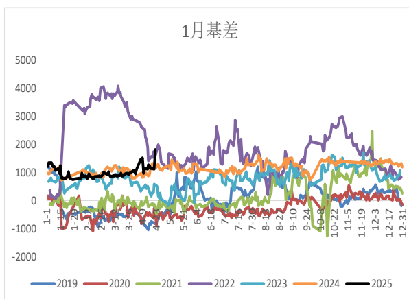
图 2：棉花 1 月基差
