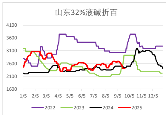
图 2：山东 32%碱现货价格
