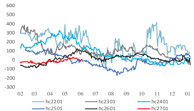
图4: 热卷01合约基差 (上海地区) (元/吨)
