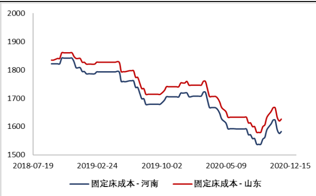
图10: 固定床工艺成本估算
