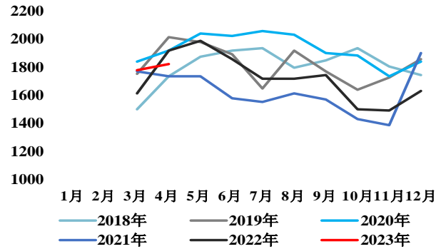
图34: 河北省生铁月度产量 (万吨)
