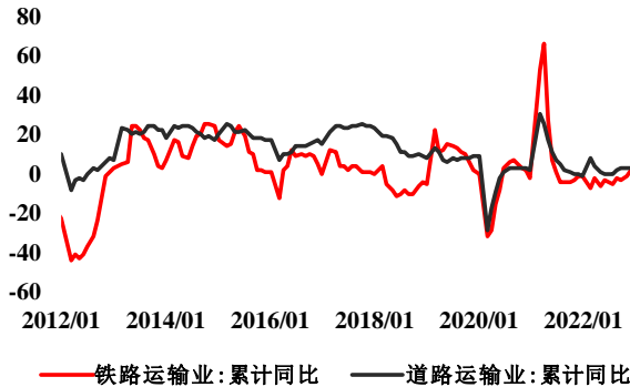
图21: 铁路、道路运输累计同比 (%)
