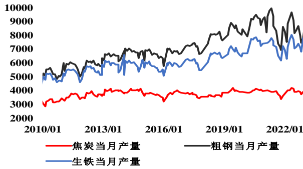
图1: 粗钢、生铁、焦炭月度产量 (万吨)
