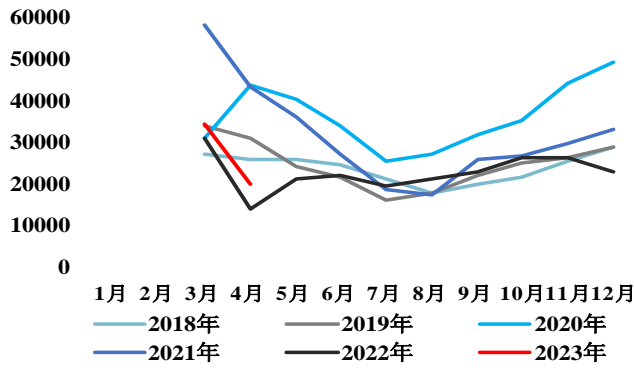
图43: 挖掘机单月产量 (台)
