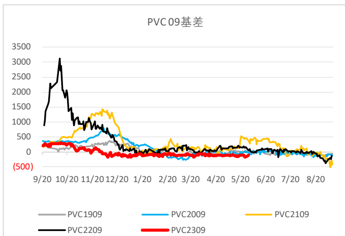
图3: PVC 基差走势
